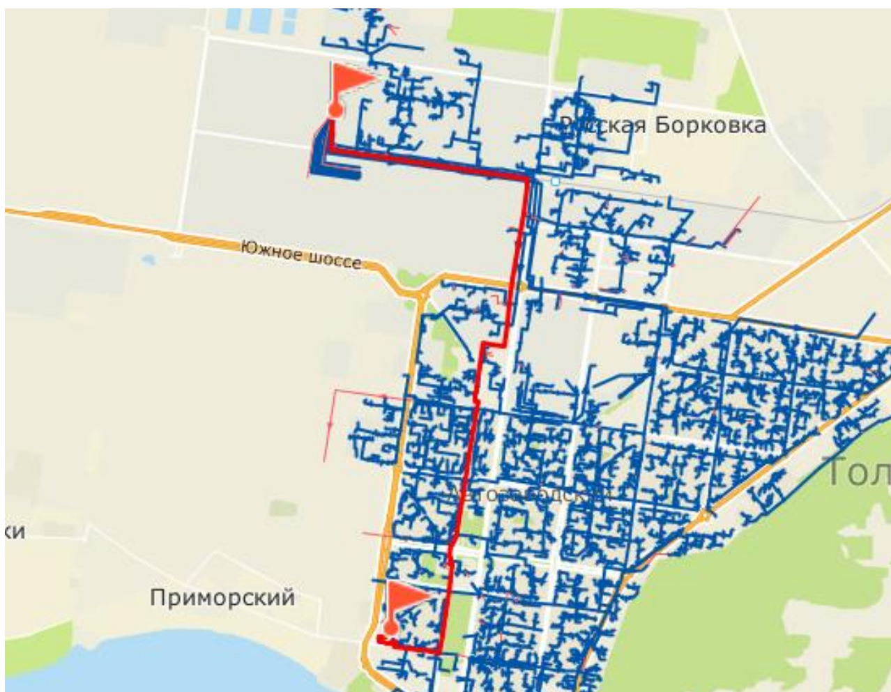
Рисунок 2.7 - Путь теплоносителя по направлению от ТЭЦ ВАЗ до потребителя «Московский пр., 59»
