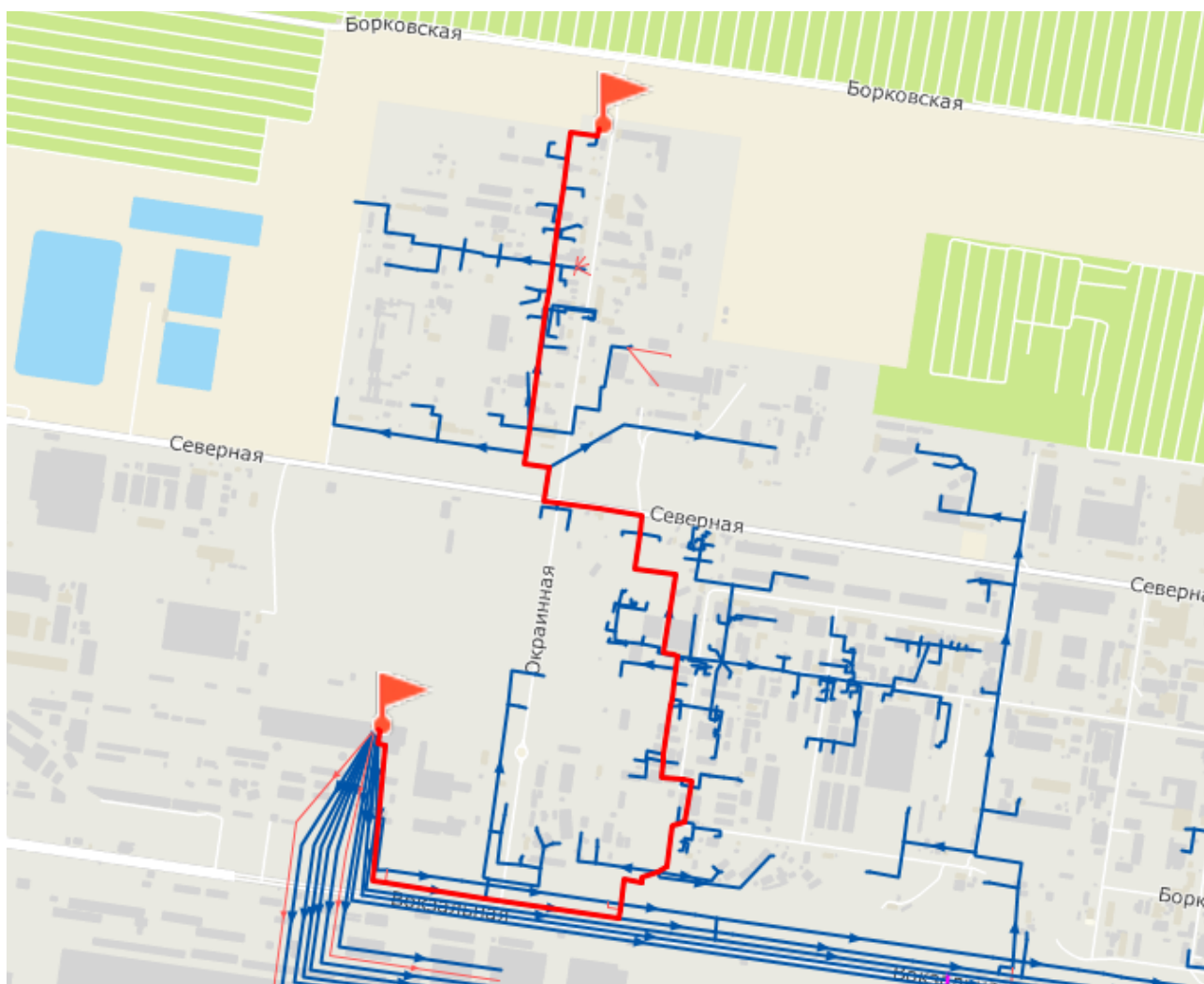
Рисунок 2.3 - Путь теплоносителя по направлению от ТЭЦ ВАЗ до потребителя «ул.Окраинная 1»
