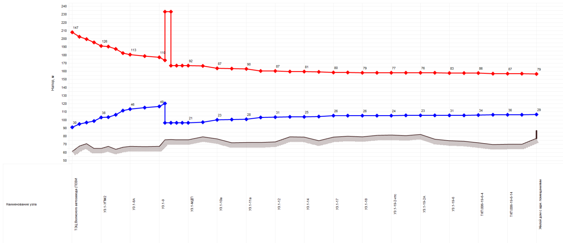
Рисунок 2.8 - Пьезометрический график от ТЭЦ ВА3 до потребителя «Московский пр., 59»
