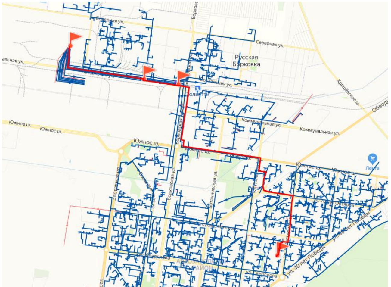
Рисунок 2.11 - Путь теплоносителя по направлению от ТЭЦ ВА3 до потребителя «ул. Автостроителей 84а»
