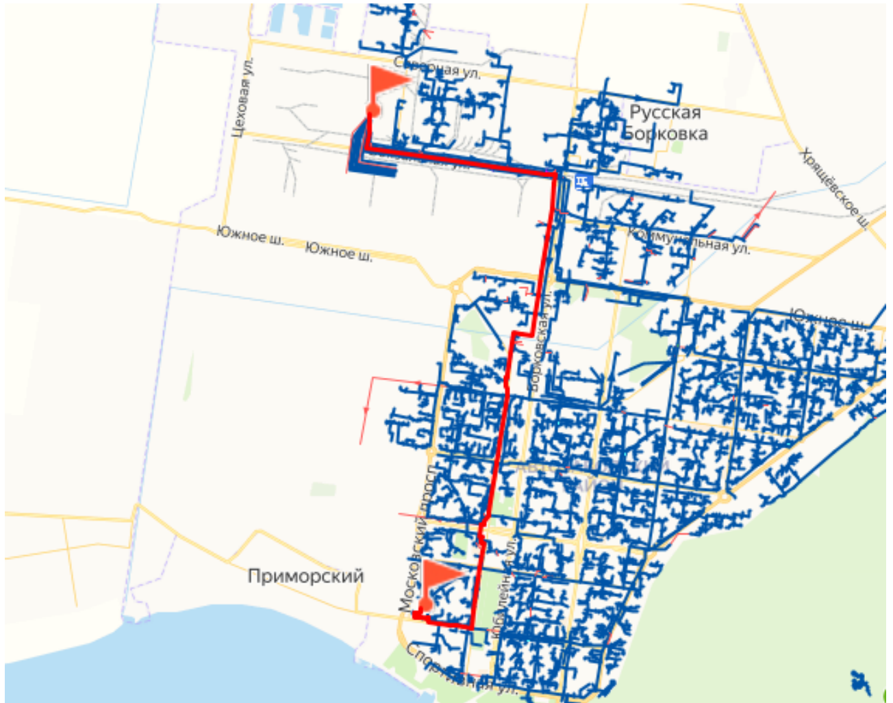
Рисунок 2.7 - Путь теплоносителя по направлению от ТЭЦ ВА3 до потребителя «Московский пр., 59»
