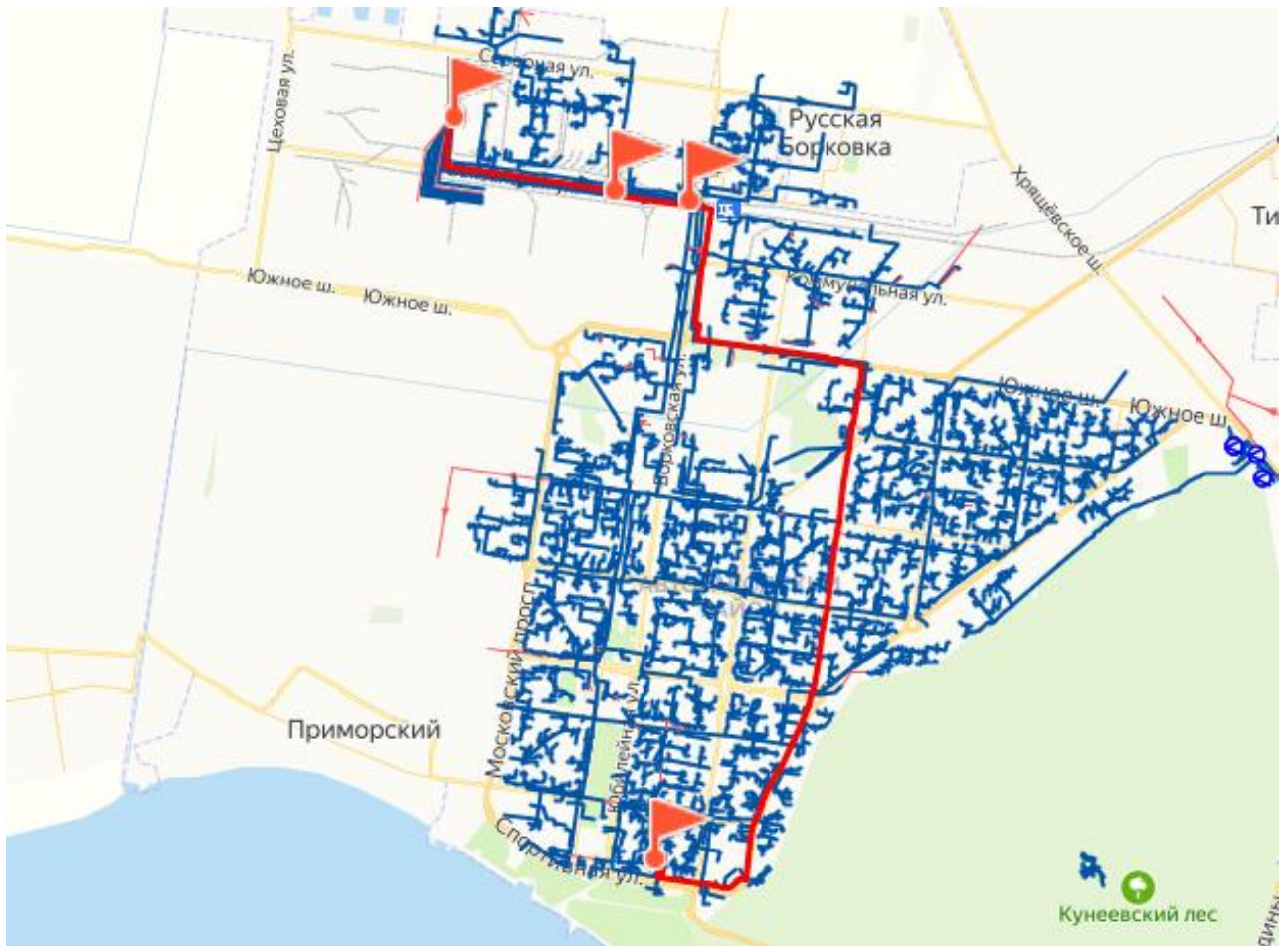
Рисунок 2.9 - Путь теплоносителя по направлению от ТЭЦ ВА3 до потребителя «ул. Спортивная 10»
