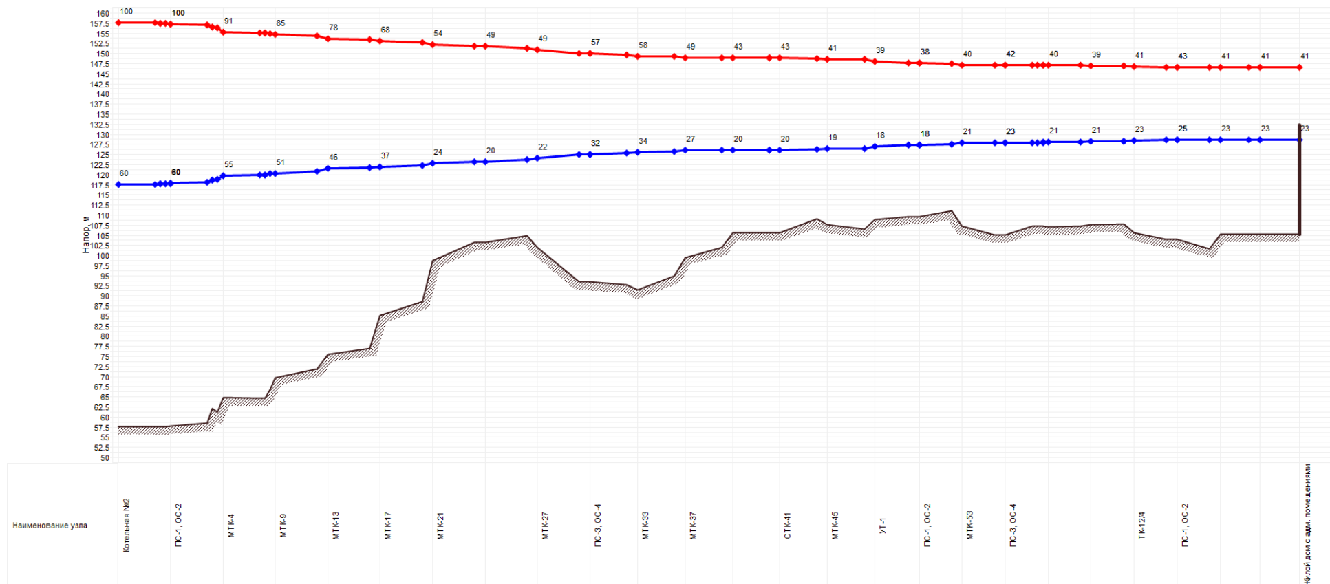
Рисунок 2.22 - Пьезометрический график от Котельной №2 до потребителя «ул. Коммунистическая 13»
