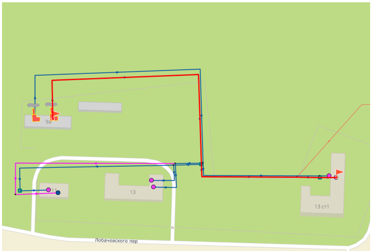
Рисунок 2.29 - Путь теплоносителя по направлению от Котельной № 7 до потребителя «ул. Лобачевского 13»
