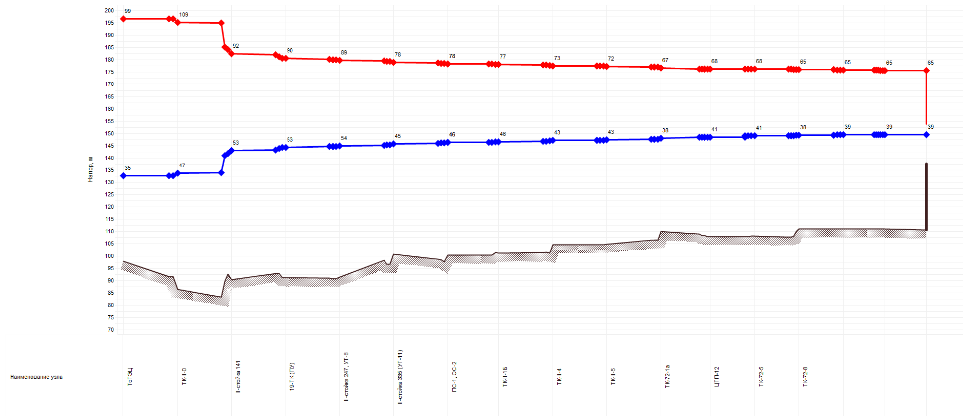
Рисунок 2.16 - Пьезометрический график от Тольяттинской ТЭС до потребителя «ул. Голосова 44»
