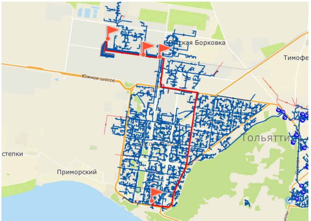
Рисунок 2.9 - Путь теплоносителя по направлению от ТЭЦ ВА3 до потребителя «ул. Спортивная 10»
