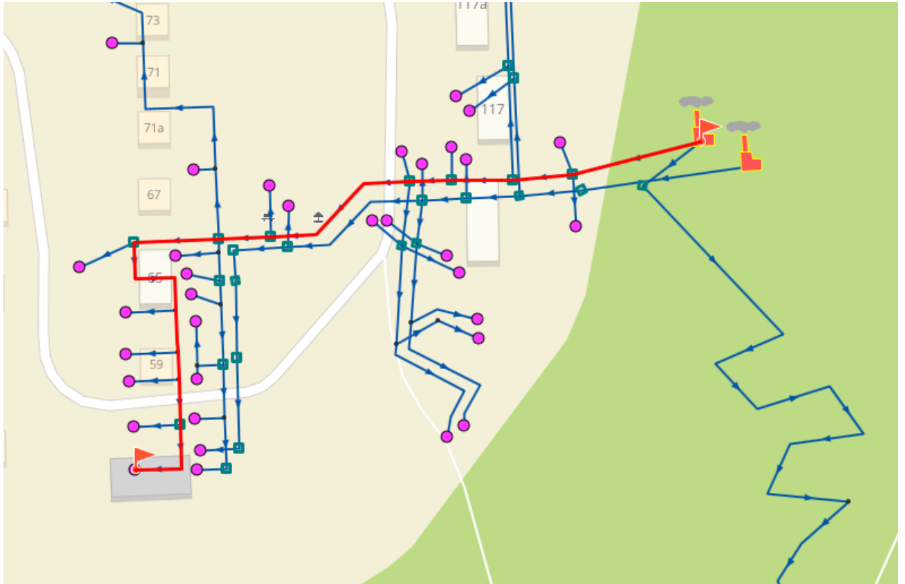
Рисунок 2.27 - Путь теплоносителя по направлению от Котельной №3 до потребителя «ул.Санаторная 55»
