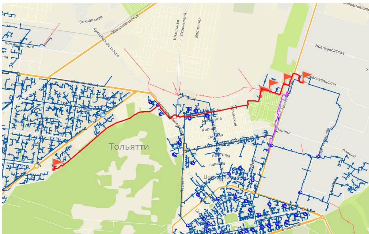
Рисунок 2.13 - Путь теплоносителя по направлению от Тольяттинской ТЭЦ до потребителя «ул. 40 лет Победы 61А»
