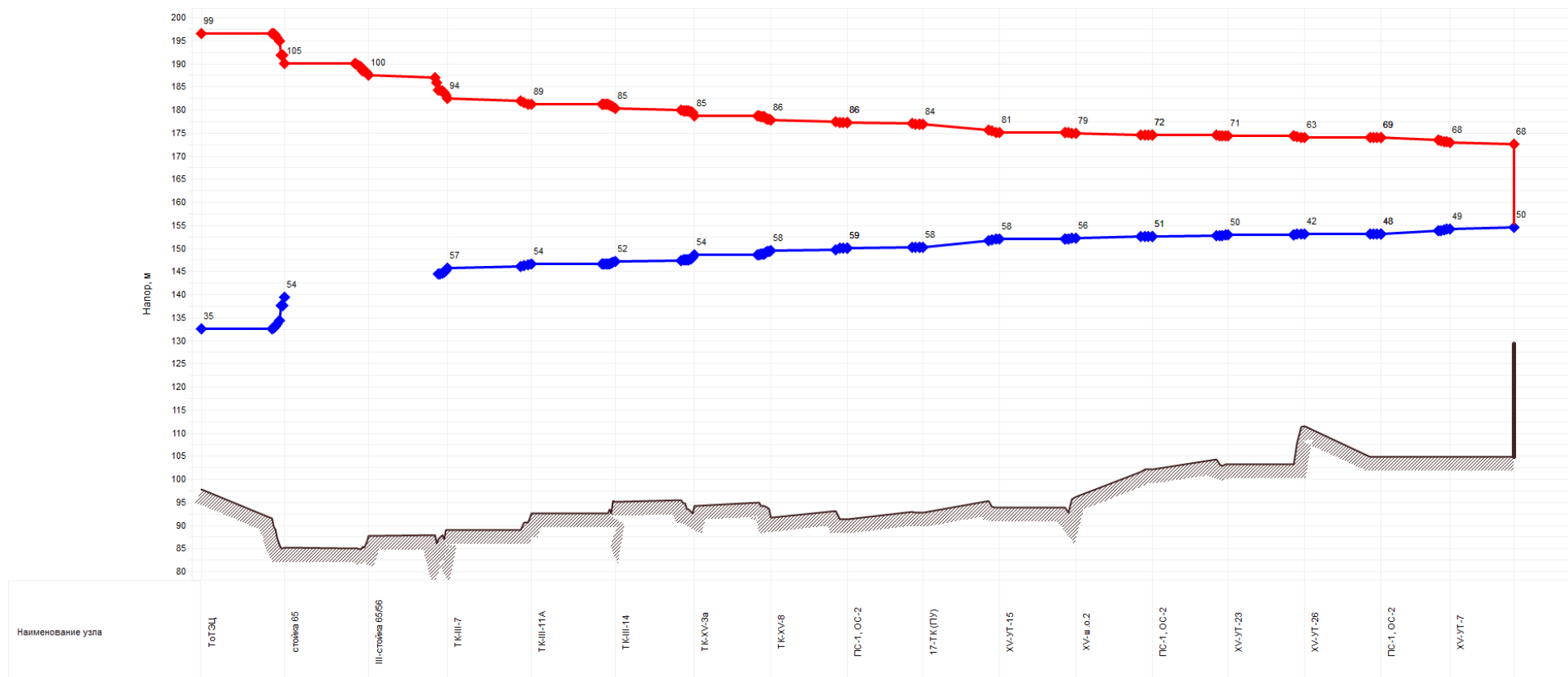
Рисунок 2.14 - Пьезометрический график от Тольяттинской ТЭС до потребителя «ул. 40 лет Победы 61А»
