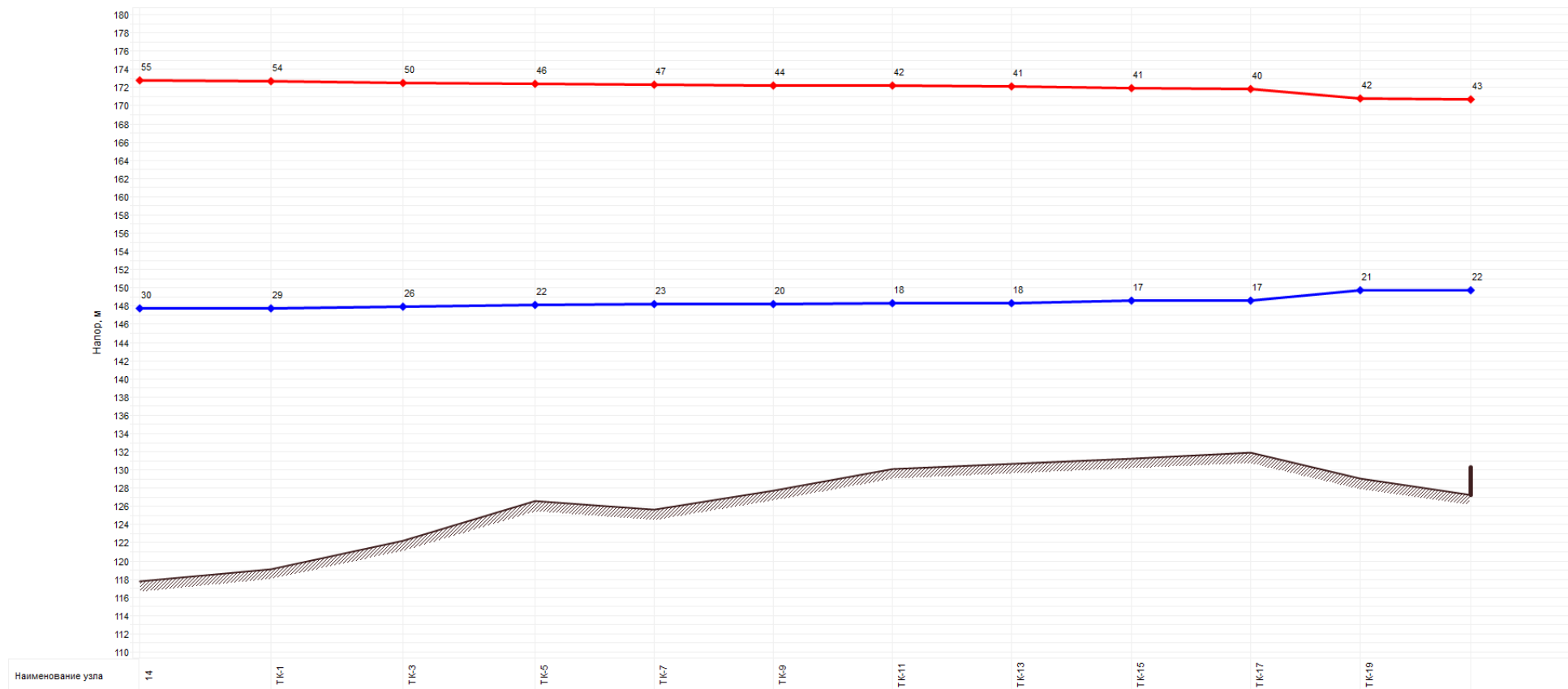
Рисунок 2.38 - Пьезометрический график от котельной № 14 до потребителя «Комсомольское шоссе 226»
