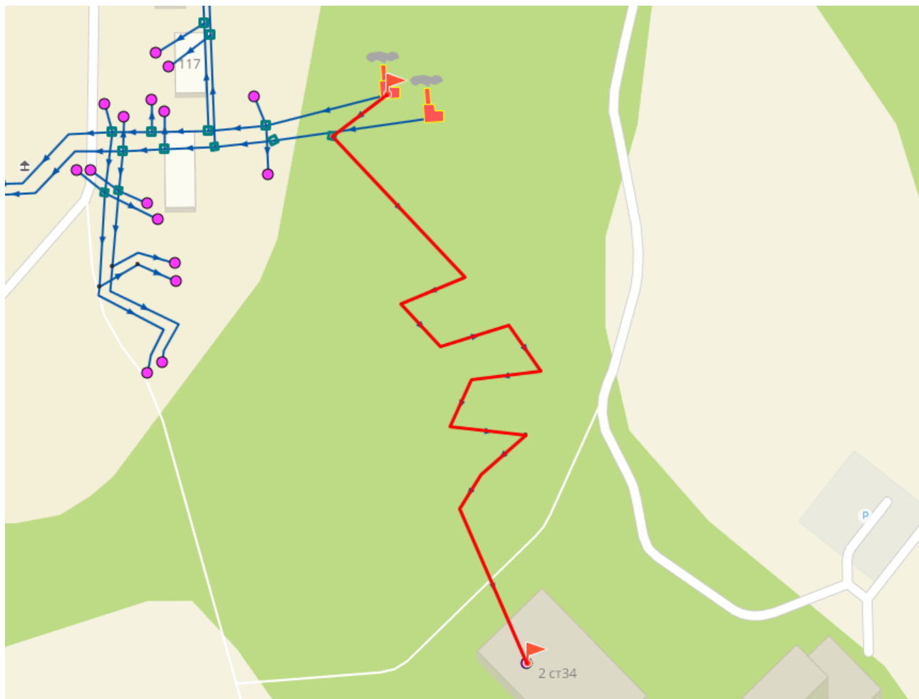
Рисунок 2.25 - Путь теплоносителя по направлению от Котельной №3 до потребителя «Лесопарковое шоссе 2»
