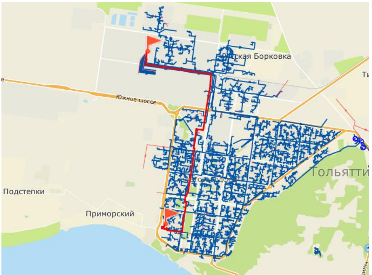
Рисунок 2.7 - Путь теплоносителя по направлению от ТЭЦ ВА3 до потребителя «Московский пр., 59»
