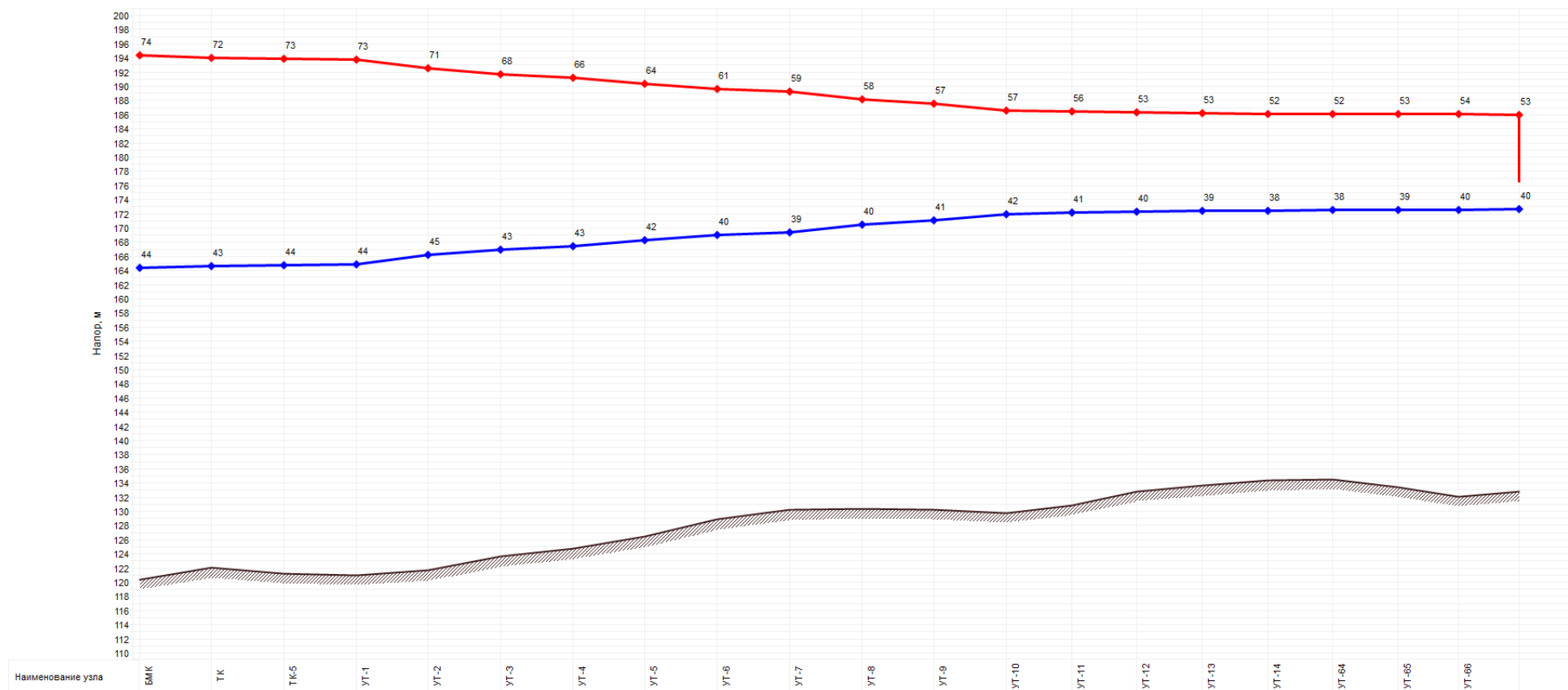
Рисунок 2.40 - Пьезометрический график от котельной от котельной БМК до потребителя «ул. Академика Скрябина 4»
