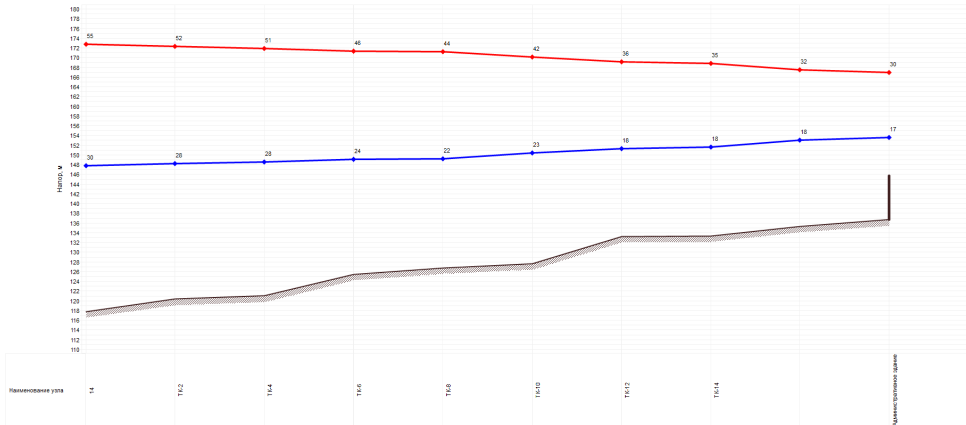
Рисунок 2.36 - Пьезометрический график от котельной № 14 до потребителя «ул. Комзина 4»
