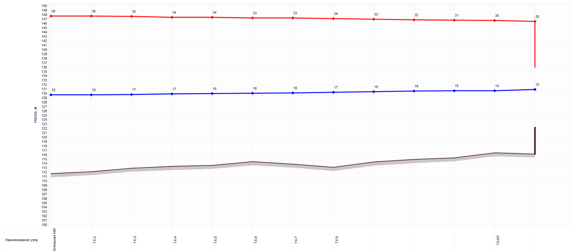
Рисунок 2.28 - Пьезометрический график от Котельной №3 до потребителя «ул. Санаторная 55»
