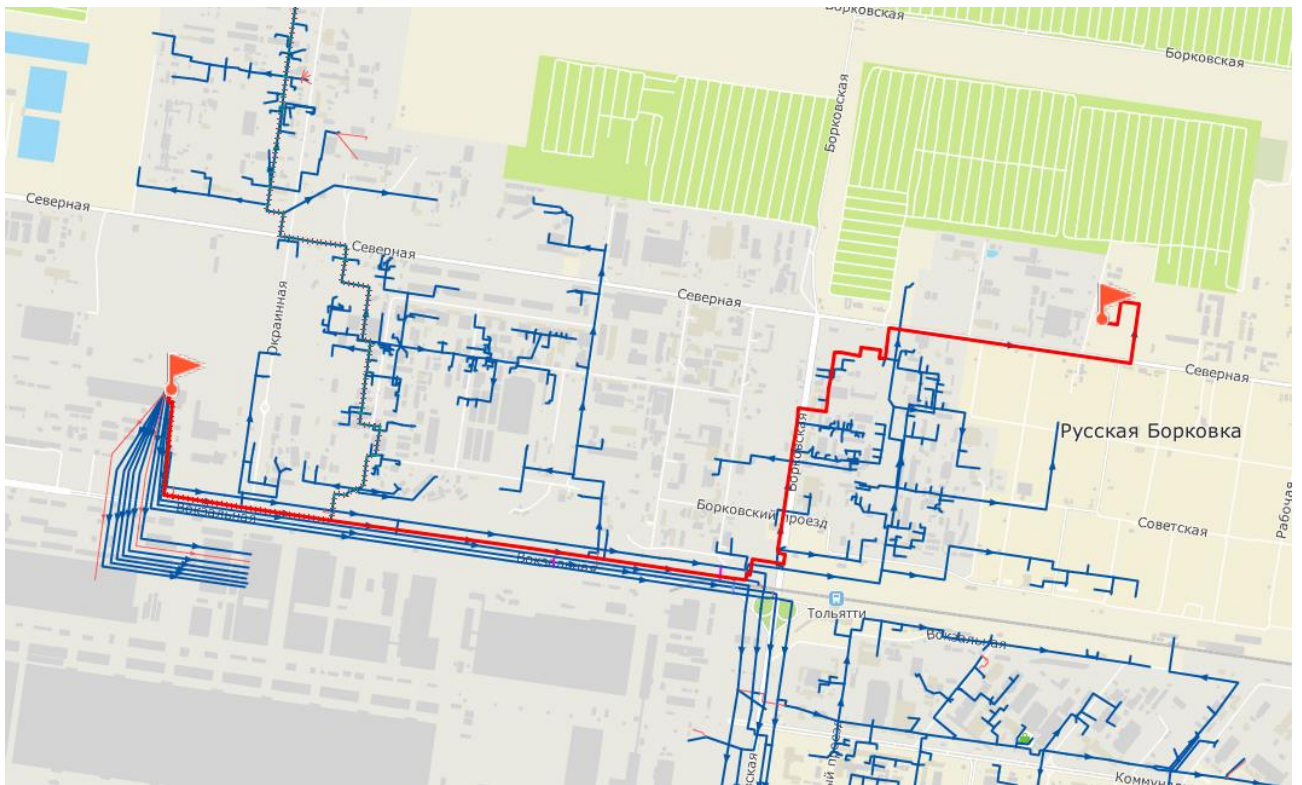
Рисунок 2.5 - Путь теплоносителя по направлению от ТЭЦ ВА3 до потребителя «ул. Северная 10»
