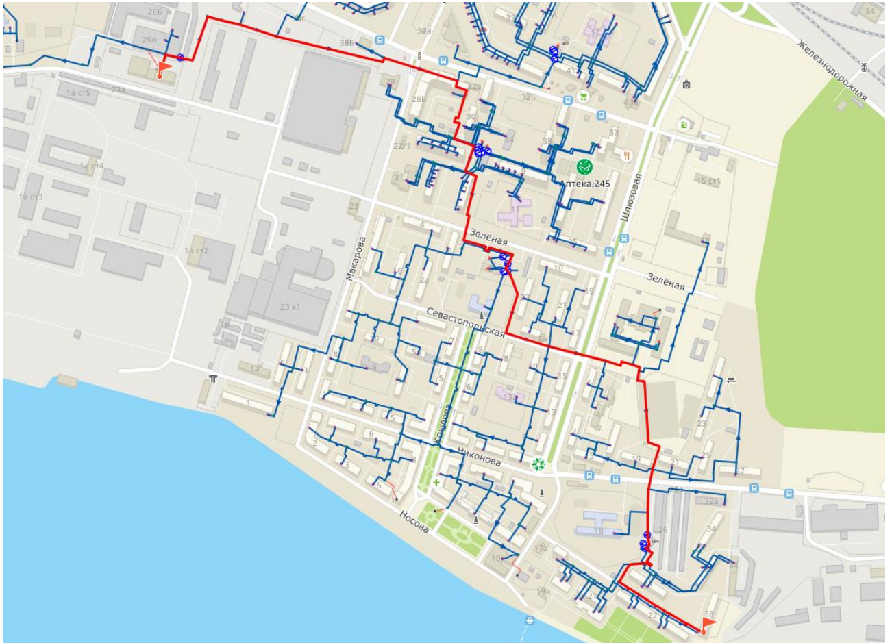
Рисунок 2.33 - Путь теплоносителя по направлению от котельной № 8 до потребителя «ул. Никонова 38»
