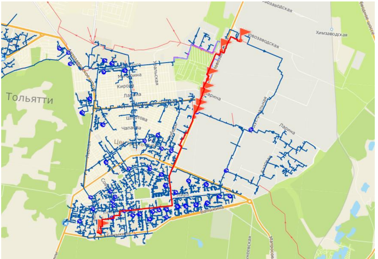
Рисунок 2.19 - Путь теплоносителя по направлению от Тольяттинской ТЭЦ до потребителя «ул. Ушакова 62»
