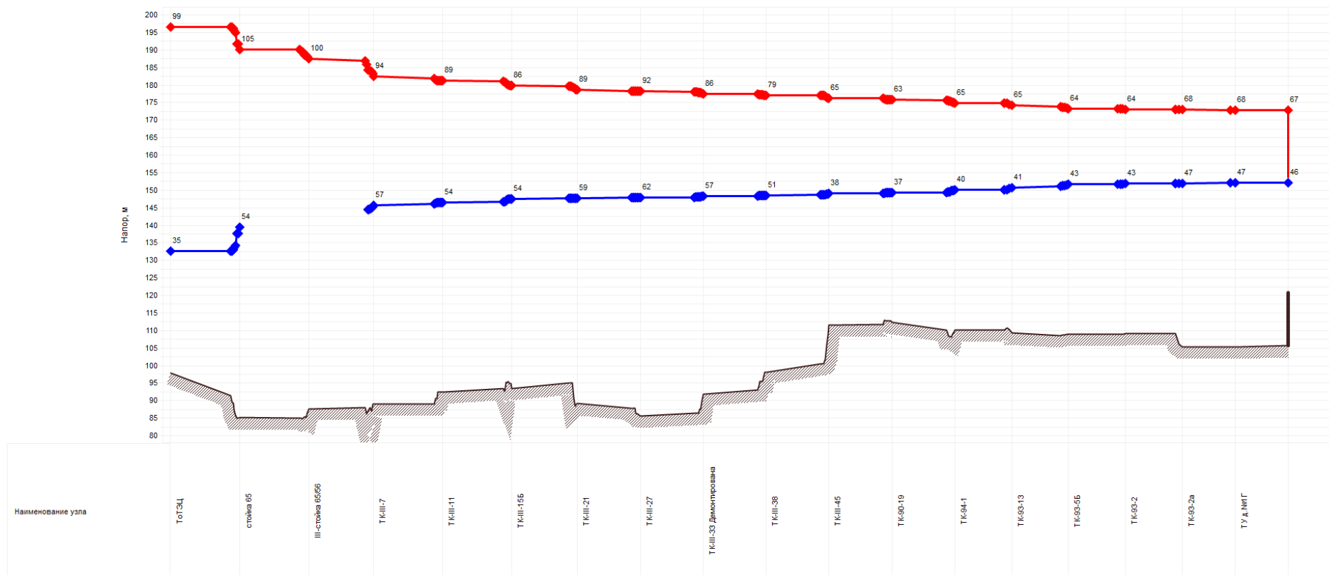
Рисунок 2.18 - Пьезометрический график от Тольяттинской ТЭЦ до потребителя «ул. Родины 1д»
