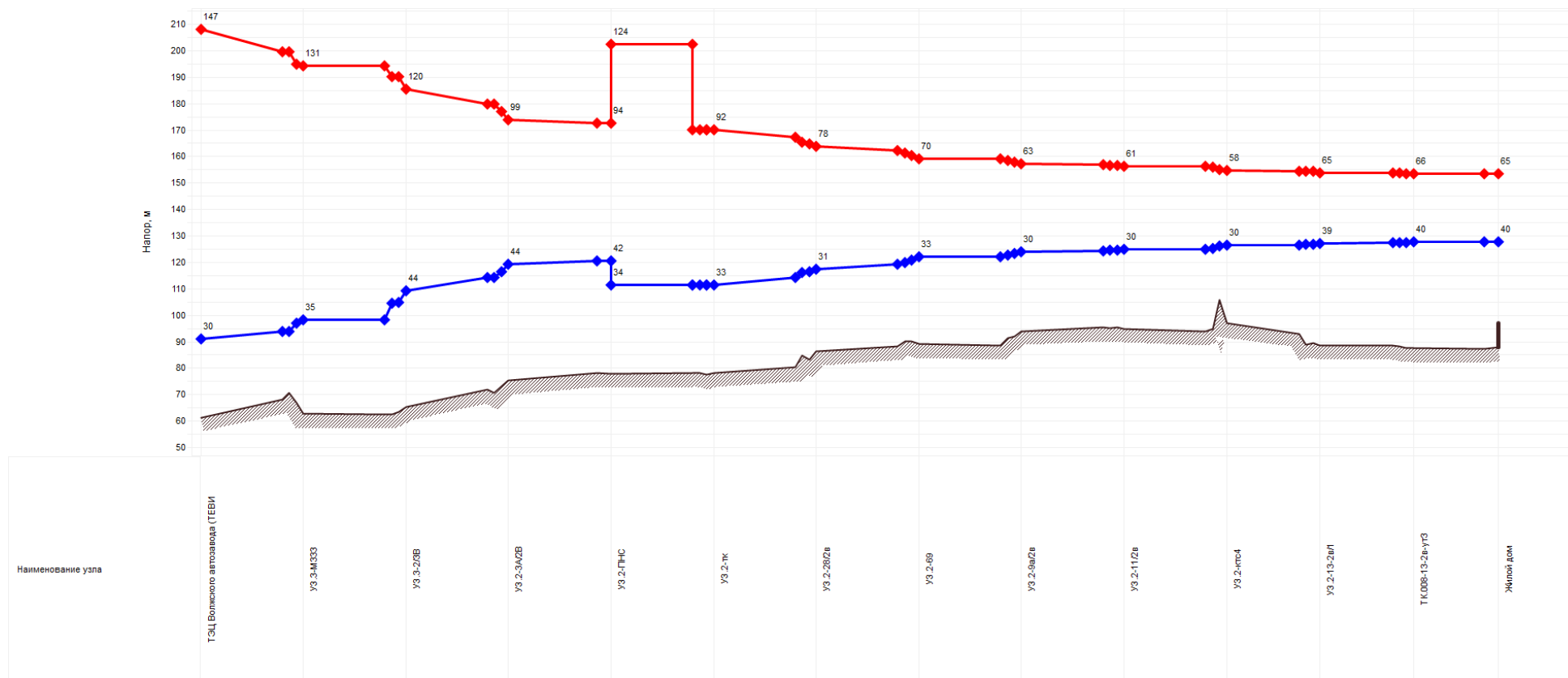
Рисунок 2.10 - Пьезометрический график от ТЭЦ ВА3 до потребителя «ул. Спортивная 10»
