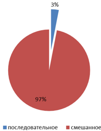
Рисунок 3.10– Типы присоединения систем ГВС к тепловым сетям ТoTC в Центральном районе
