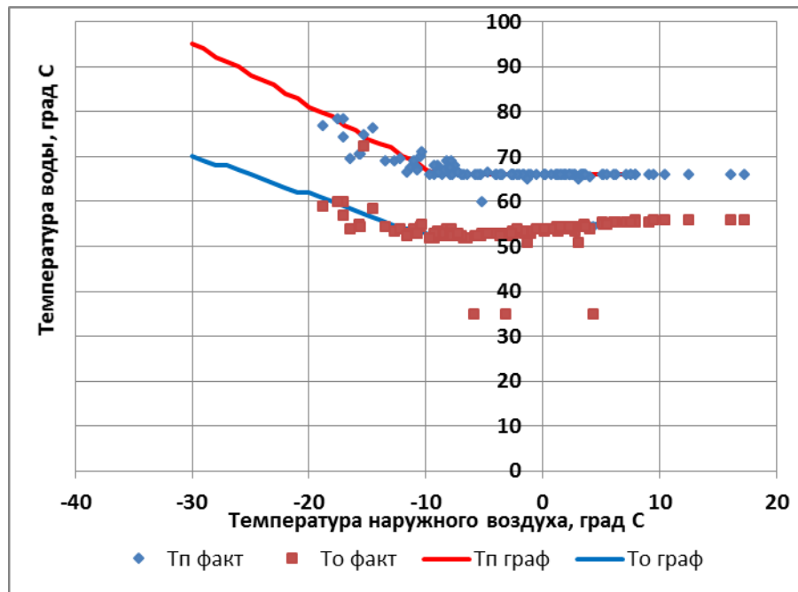
Рисунок 5.18 – Температурный график и температура сетевой воды котельной №4
