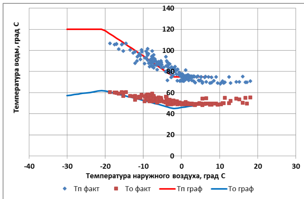
Рисунок 5.2 – Температурный график и температура сетевой воды ТпТЭЦ на «Завод ТП-1»
