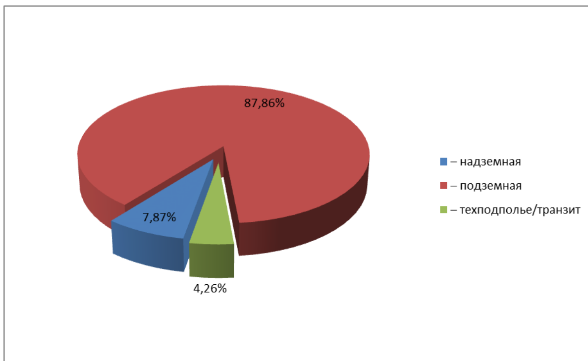
Рисунок 1.3 - Распределение суммарной протяженности водяных тепловых сетей по способам прокладки
