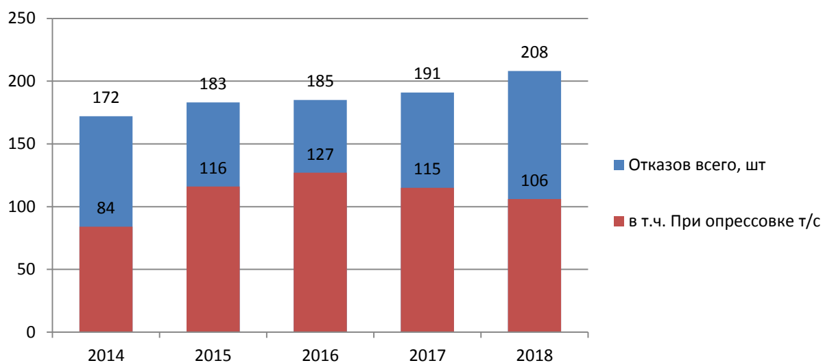
Рисунок 4 – Динамика отказов тепловых сетей ОАО «ТЕВИС» (Автозаводской район) за период 2014-2018 гг.
